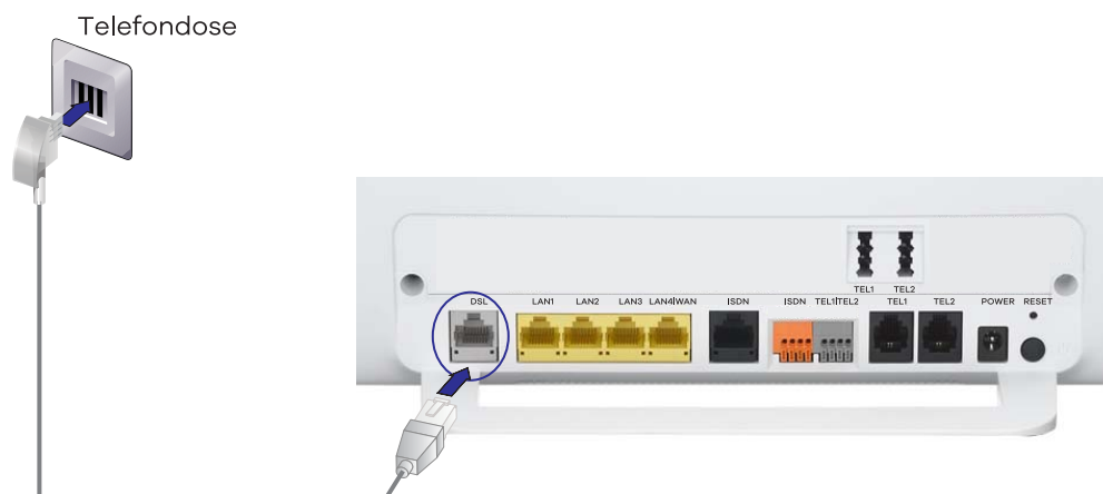
Abbildung 1 IP-basierender Breitbandanschluss
