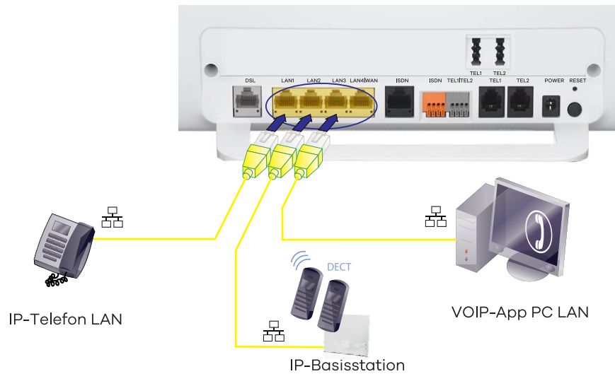
Abbildung 4 IP-Telefone anschließen
