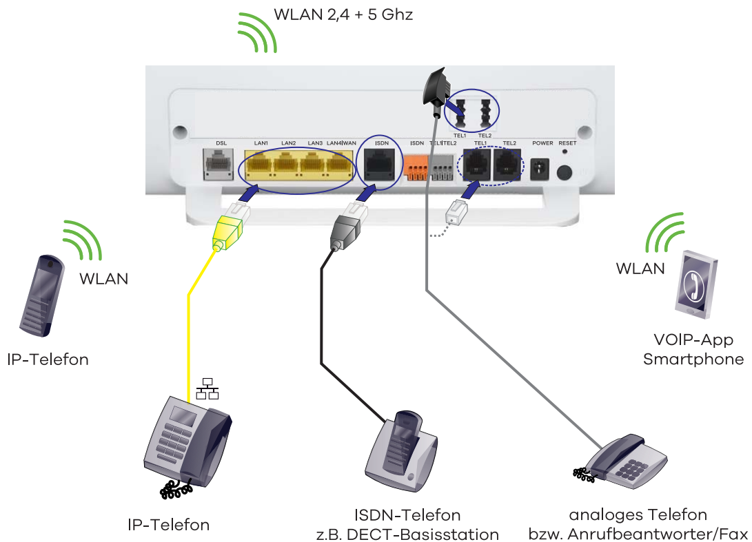
Abbildung 3 Digitalisierungsbox BASIC als Telefonanlage (PBX)
