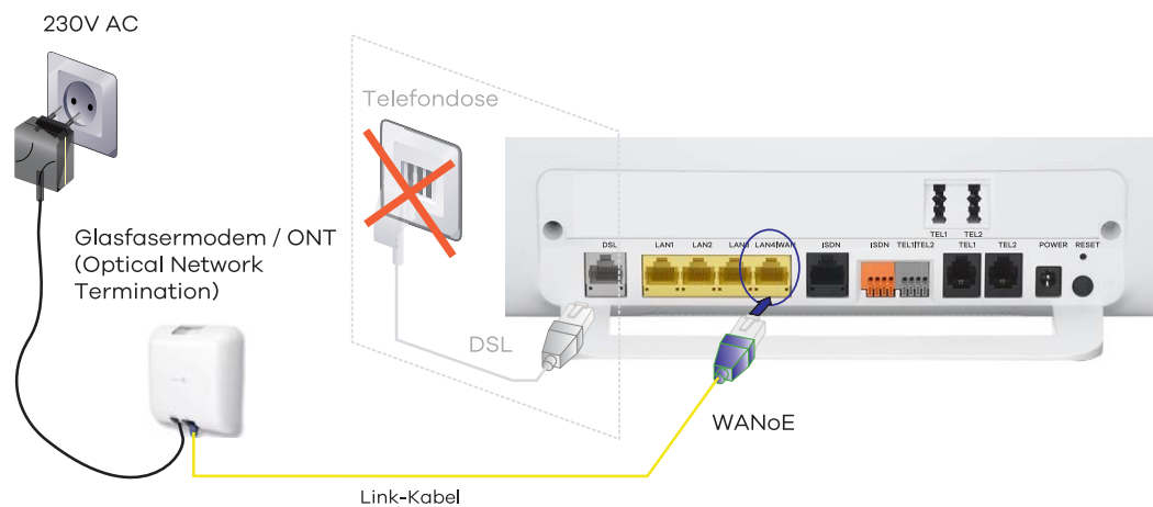
Abbildung 2 Anschlussvariante WAN over Ethernet
