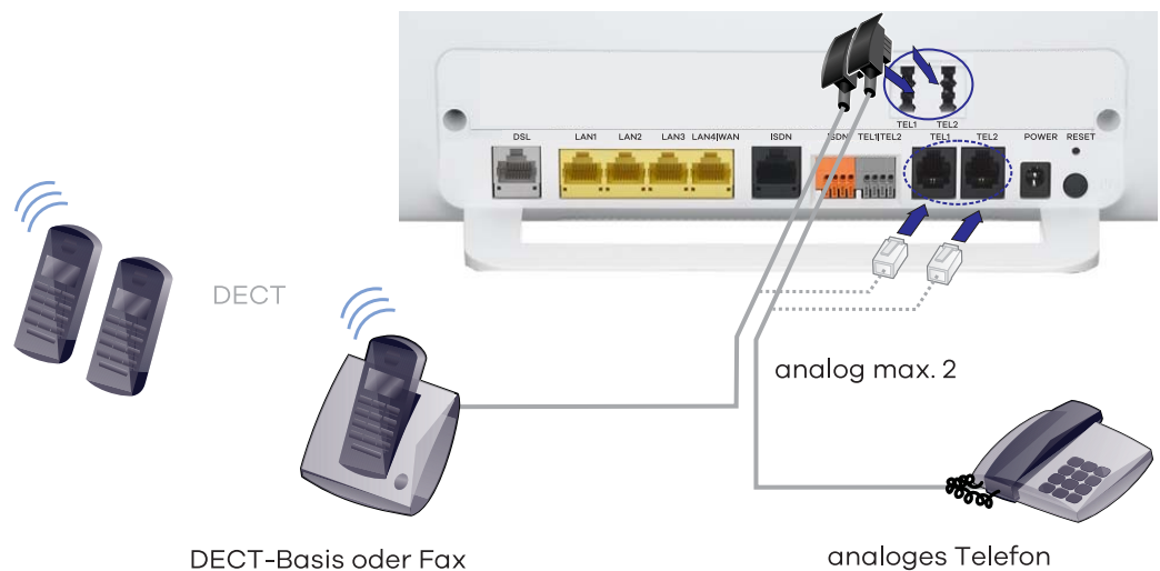
Abbildung 2 Analoge Telefone anschließen
