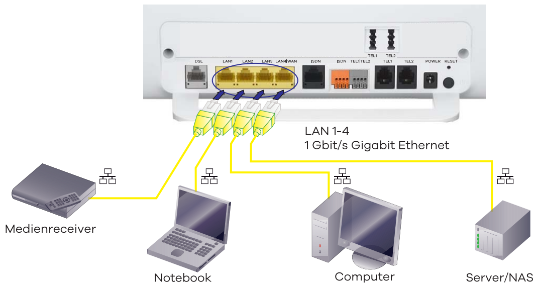
Abbildung 6 Computer anschließen
