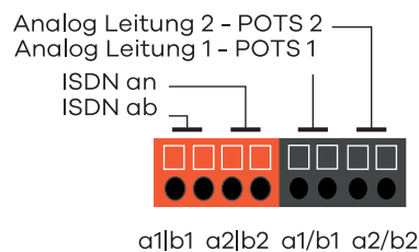
Abbildung 5 Anschlussklemmen für Direktverdrahtung
