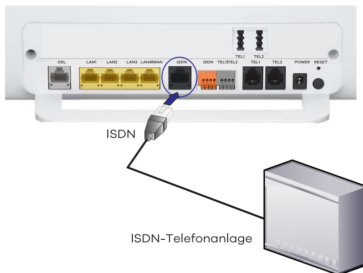
Abbildung 9 ISDN-Telefonanlage verwenden
