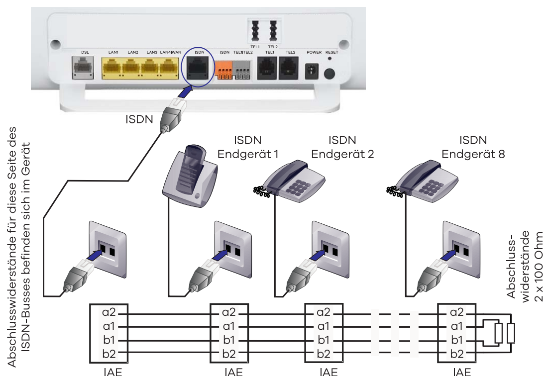
Abbildung 8 Verbindung mit einem ISDN-Bus herstellen
