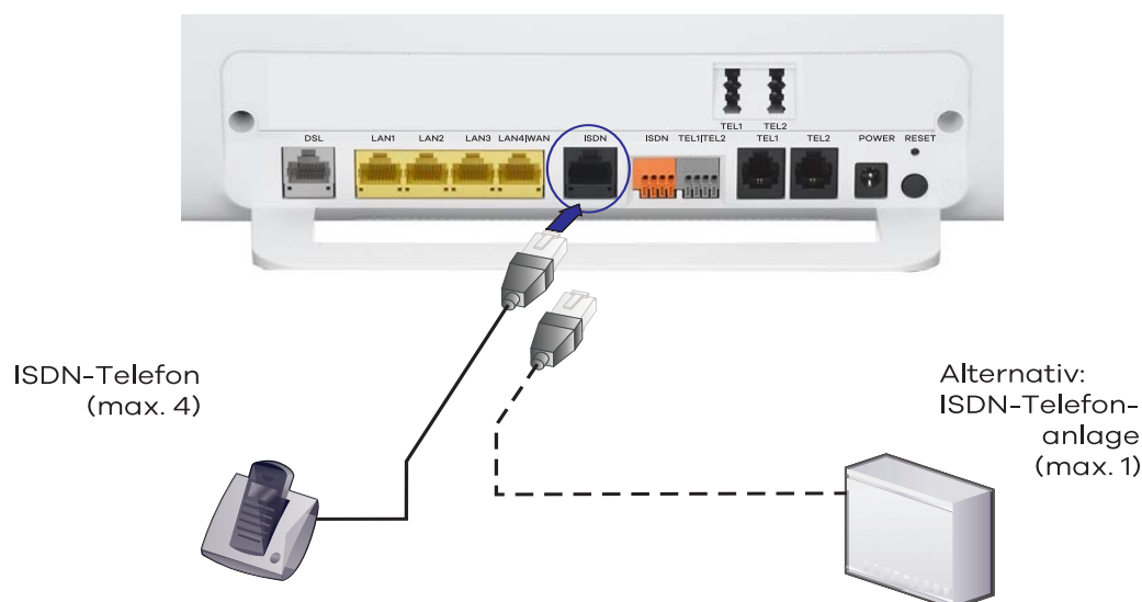
Abbildung 3 ISDN-Telefone anschließen
