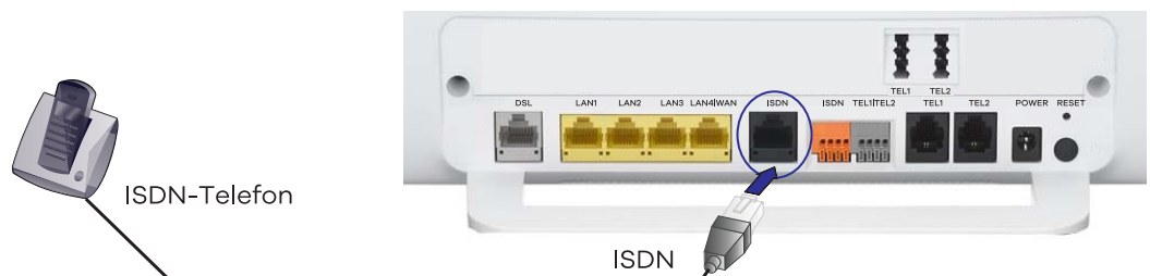
Abbildung 7 Verbindung mit einem ISDN-Gerät herstellen
