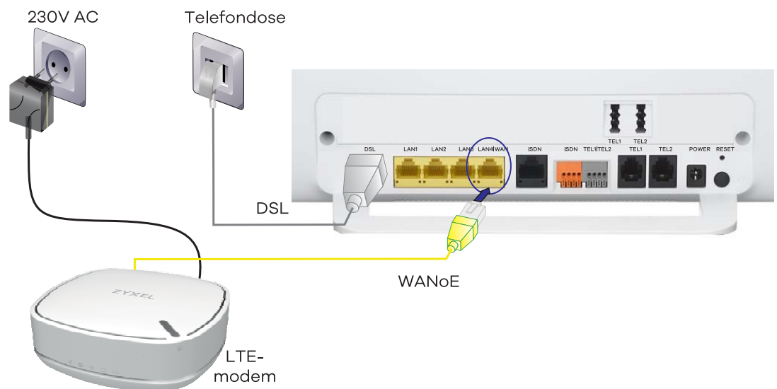
Abbildung 3 LTE-Backup
