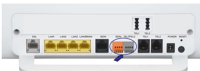
Anschlussklemmen für Direktverdrahtung
