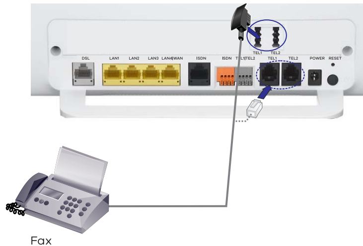
Abbildung 6 Fax verwenden
