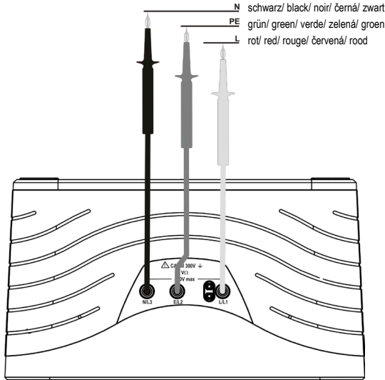
Bild 5: Spannungs-, RCD- und Zs-/ Zi-Messung über 4 mm Messleitung Figure 5: Measurement of voltage, RCD and Zs (Zloop)/Zi (Zline) via of 4 mm measuring leads Fig. 5: Mesure de tension, RCD et Zs/Zi avec des câbles de mesure de 4 mm Obr. 5: Měření napětí, RCD, Zs/Zi pomocí měřících vedení 4 mm Fig. 5: Voltage-, RCD- en Zs/Zi-meting via meetsnoeren van 4 mm
