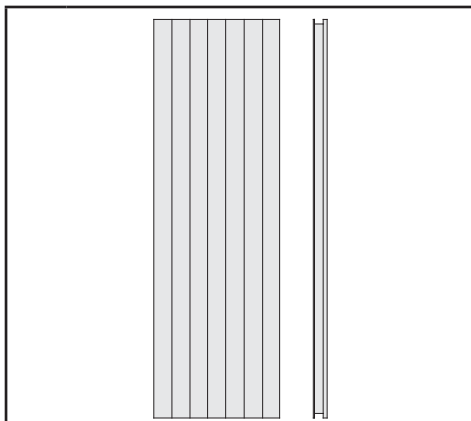
2 x W4 | 1920 x 606 x 57 mm | ID 23624
