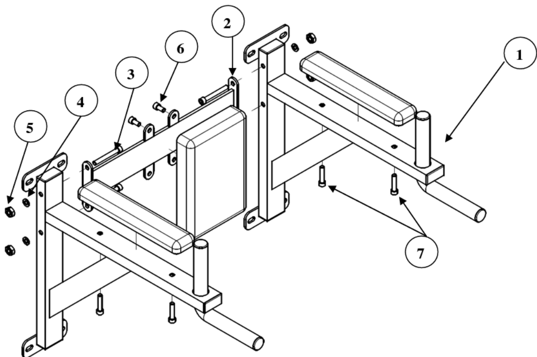
Abbildung 2: Wandhalterung für Dipstation
