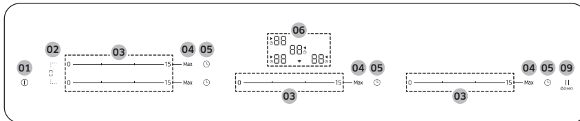
Bedienfeld 3 - NZ84C6057**
