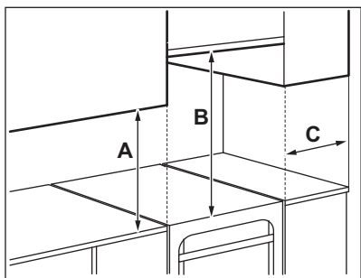
Mindestabstände
