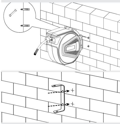
Abb. 1 Wandmontage
