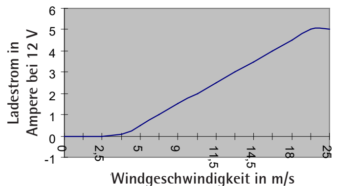
Leistungskurve „WG 504“
