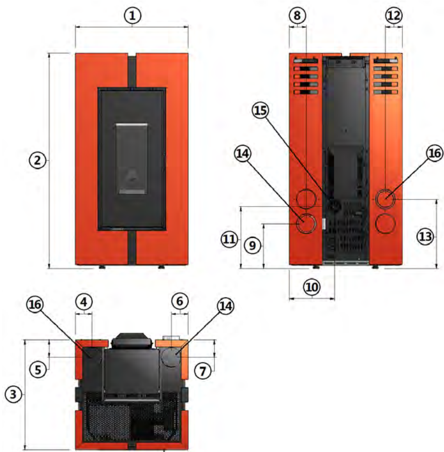
Fig. 17 - Allgemeine Abmessungen: Doge 3 Plus
