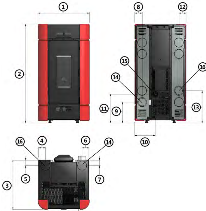
Fig. 16 - Allgemeine Abmessungen: Sire 3 Plus
