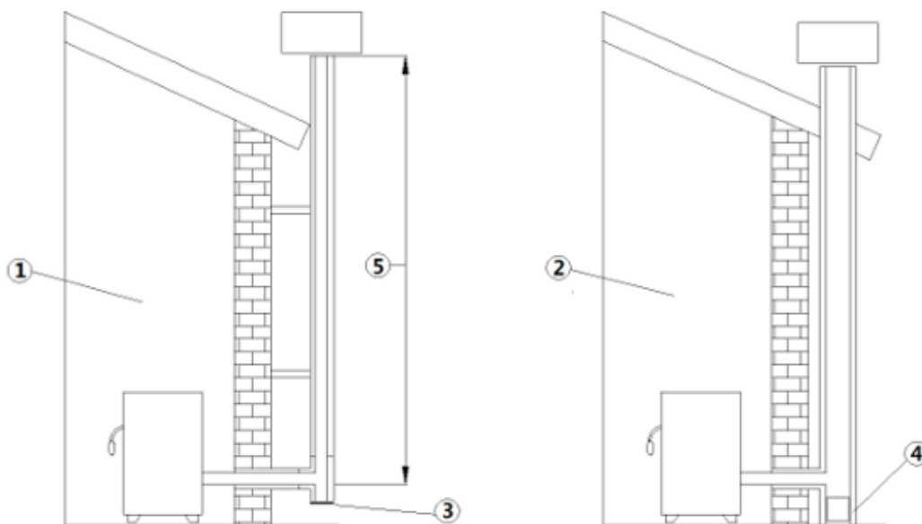
Fig. 2 - Rauchabzüge
