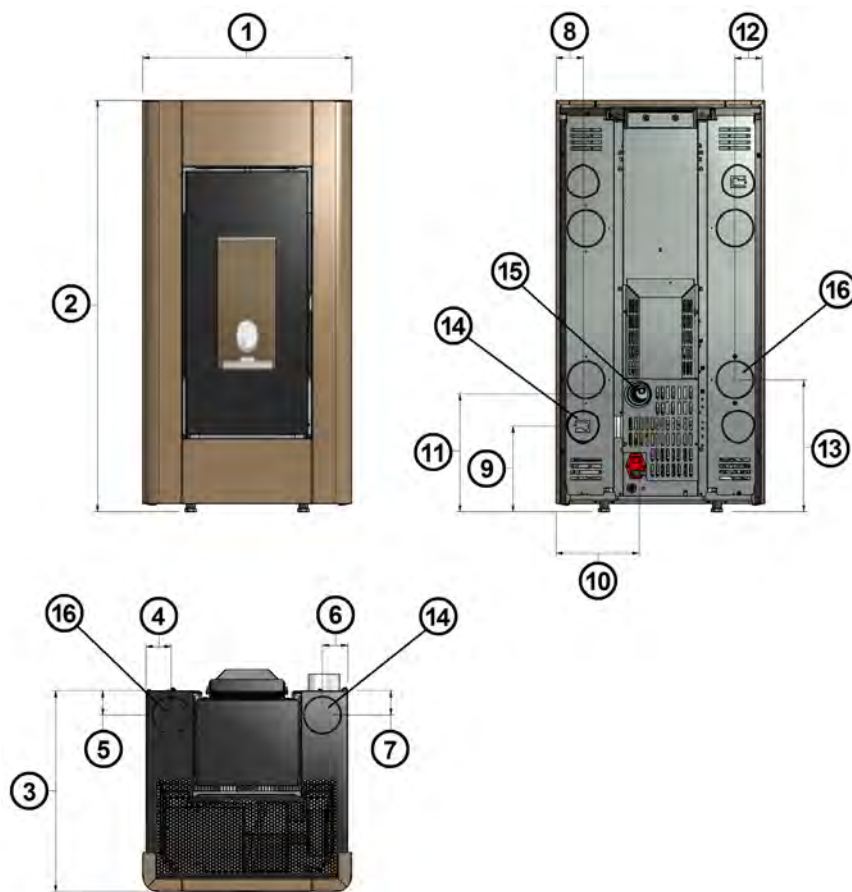
Fig. 19 - Allgemeine Abmessungen: Prince 3 / Prince 3 Plus
