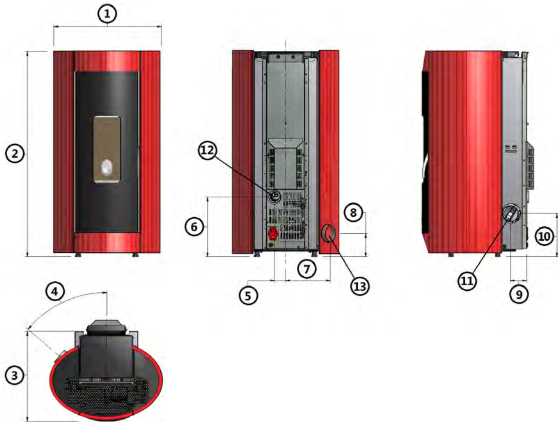
Fig. 20 - Allgemeine Abmessungen: Elise 3 Plus
