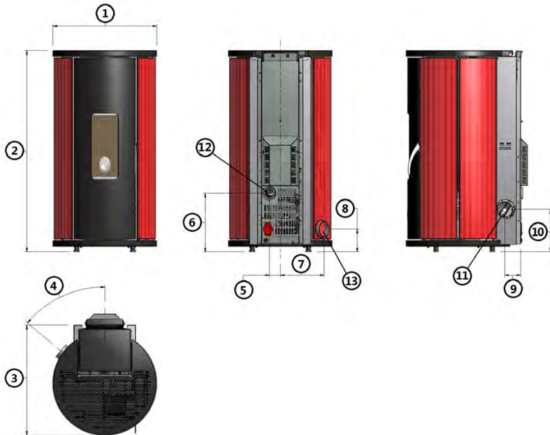
Fig. 18 - Allgemeine Abmessungen: Sfera 3 / Sfera 3 Plus / Globe
