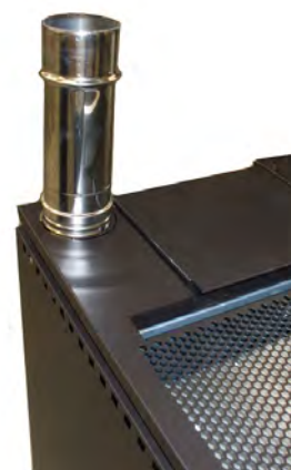
Fig. 46 - Oberer Warmluftauslass
