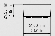
Aufputzgehäuse
