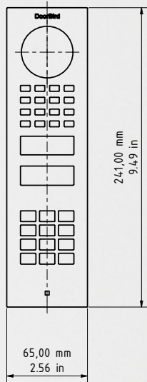
Frontblende
