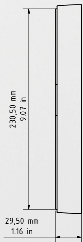
Aufputzgehäuse
