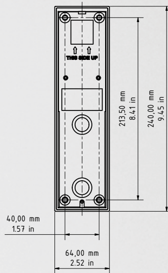
Aufputzgehäuse
