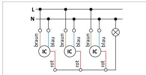
Parallelschaltung Bewegungsschalter
