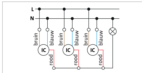
Parallele schakeling bewegingschakelaar
