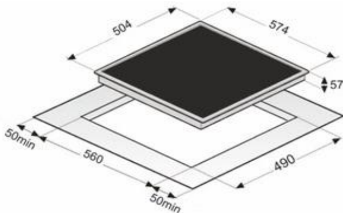
Einbauskizze
