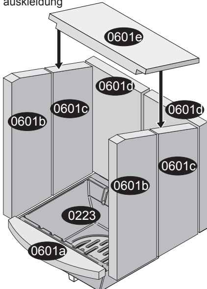
Feuerraumauskleidung
