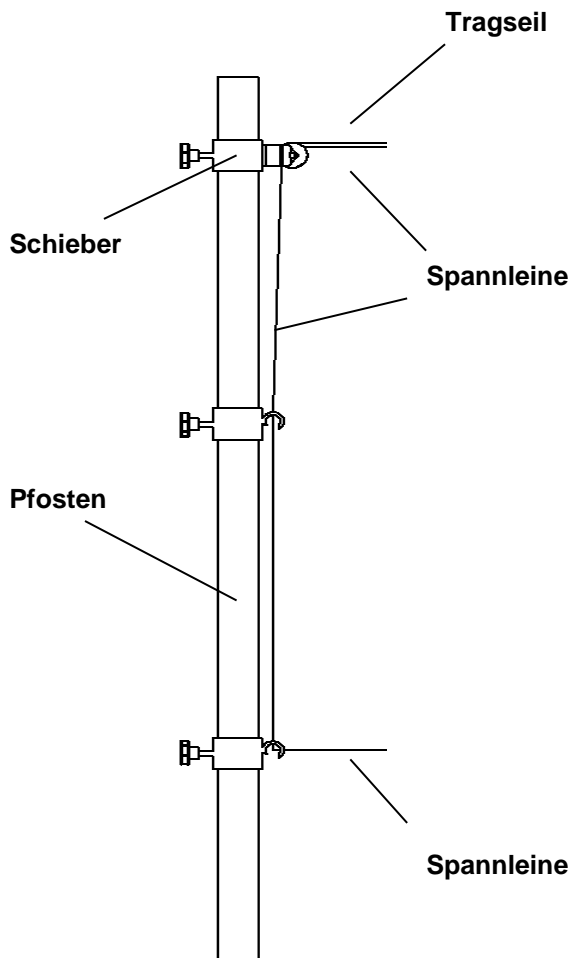
Abbildung 5: Säule mit Spannleine
