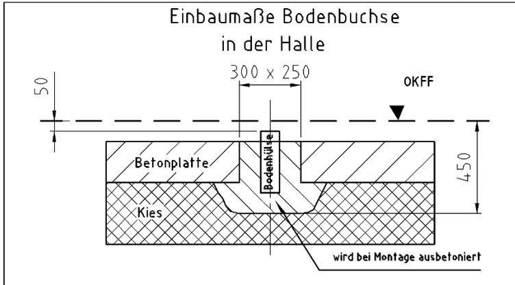
Abbildung 3: Montage Bodenhülse
