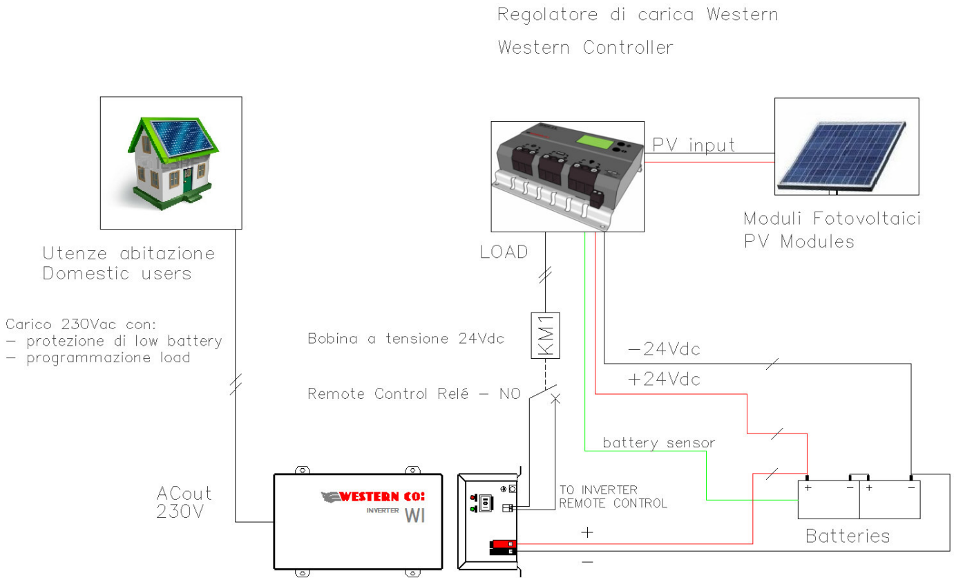
Fig. 4 Schema di collegamento WI800-24
