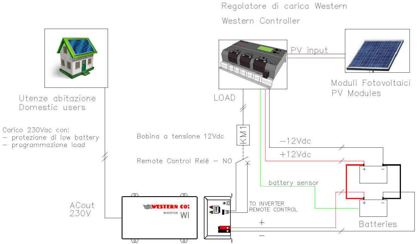
Fig. 3 Schema di collegamento WI800-12
