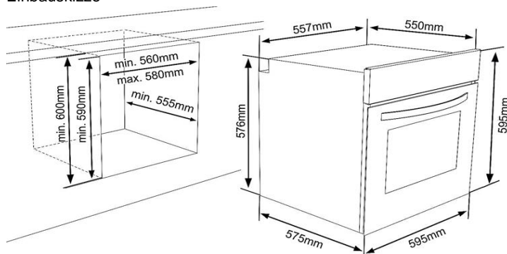
Einbauskizze
