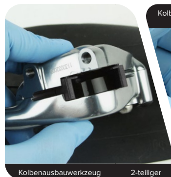
Kolbenausbauwerkzeug
