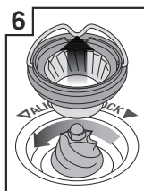
Oberen Mahlkonus entfernen
