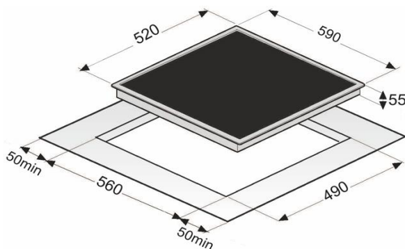
Einbauskeizze
