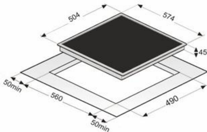
Einbauskizze
