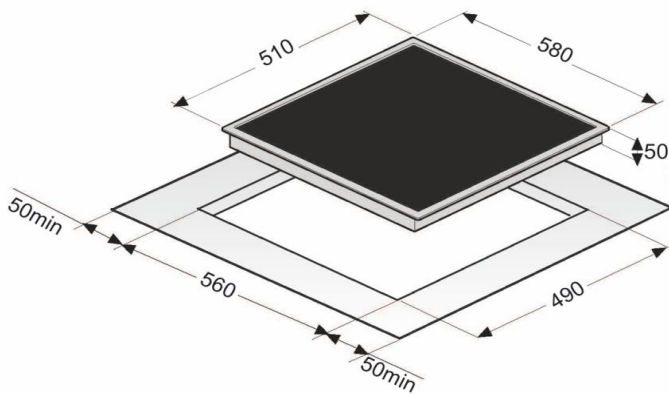
Einbauskeizze
