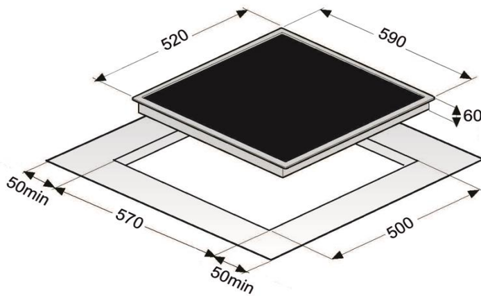
Einbauskizze
