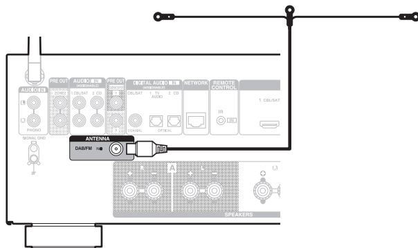
DAB-/UKW-Zimmerantenne (im Lieferumfang enthalten)
