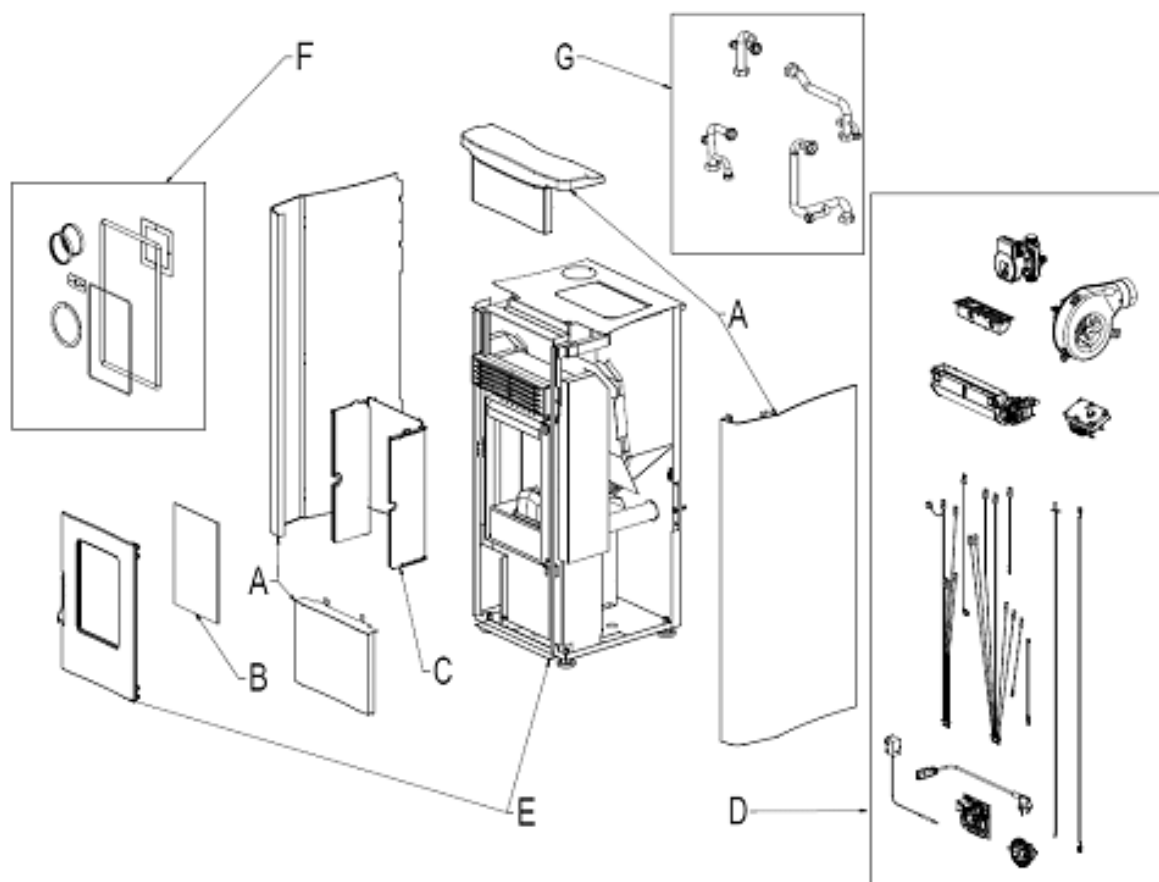
Fig. 1 - Explosionszeichnung
