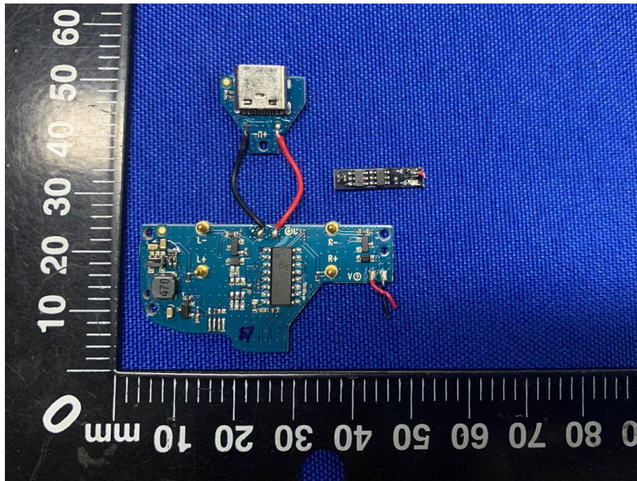
Picture 6 Front view of PCM 图6: 保护电路正面
