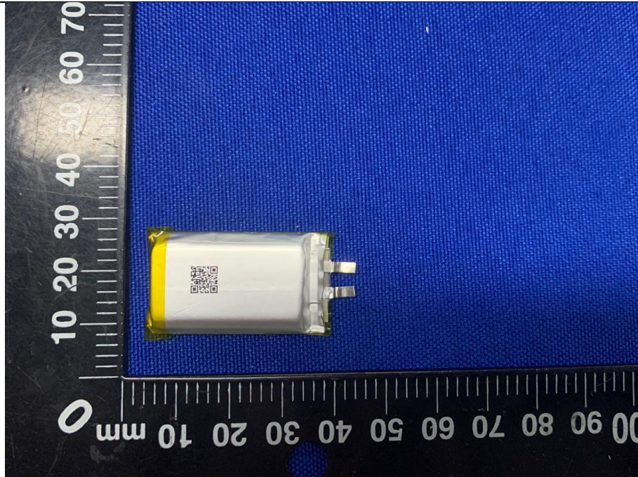
Picture 9 Back view of cell 图 9: 电芯反面
