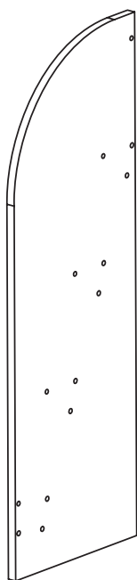
1 Seitenwand, links 1x
