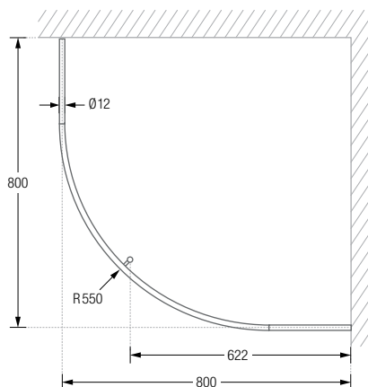
Produktbeispiel DSB550-800 Draufsicht:
