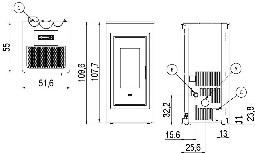
Fig. 13 - Allgemeine Abmessungen: Koba 11 - Koba Plus 11
