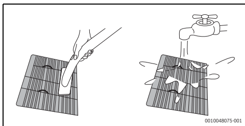
Bild 22 Reinigen des unteren und oberen Filters
