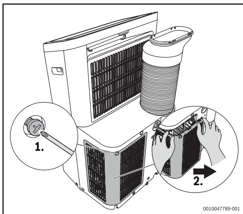
Bild 20 Demontage des unteren Filters
