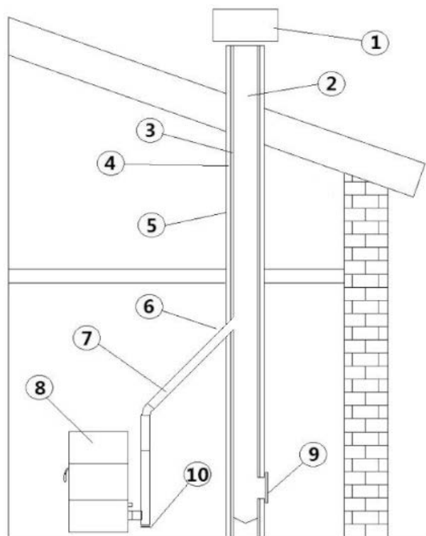
Fig. 2 - Bauteile Kamin
