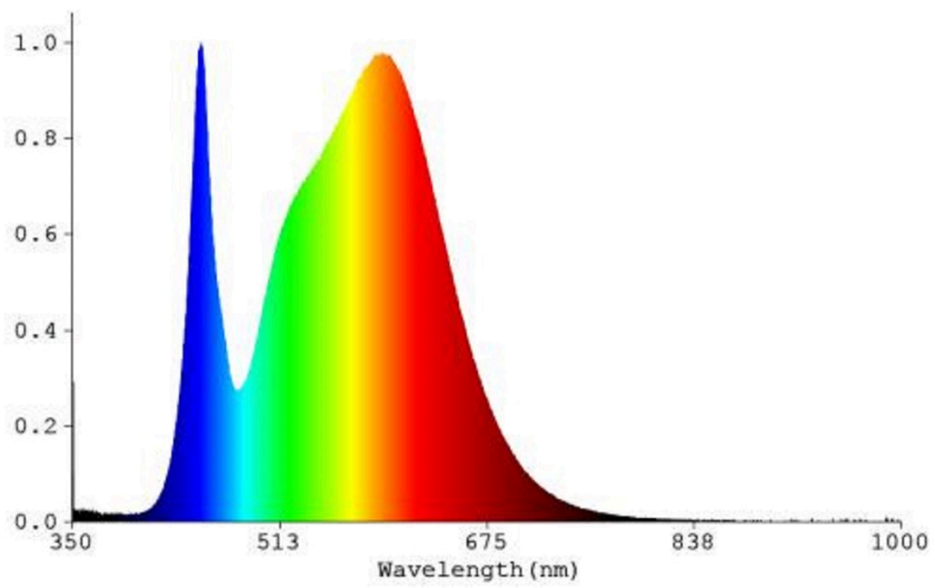
SMD2835-12C5B-0.5M-40
