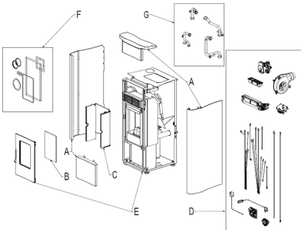
Fig. 1 - Explosionszeichnung
