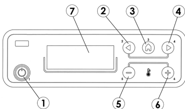
Fig. 7 - Bedientafel
