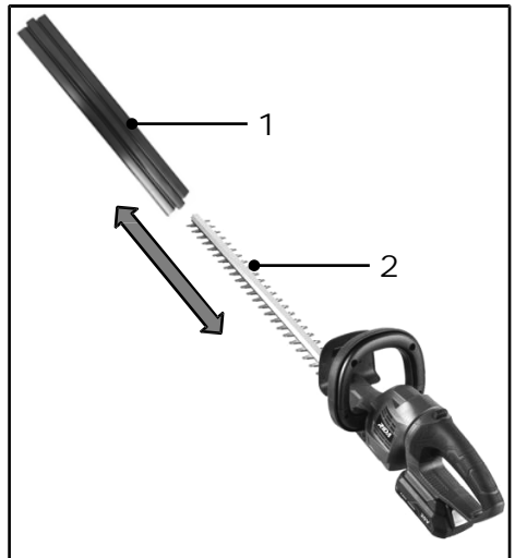
► 1. Messerschutz 2. Messerleiste
