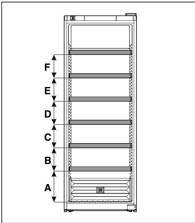
Fig. 18 Abstände Auflageroste
