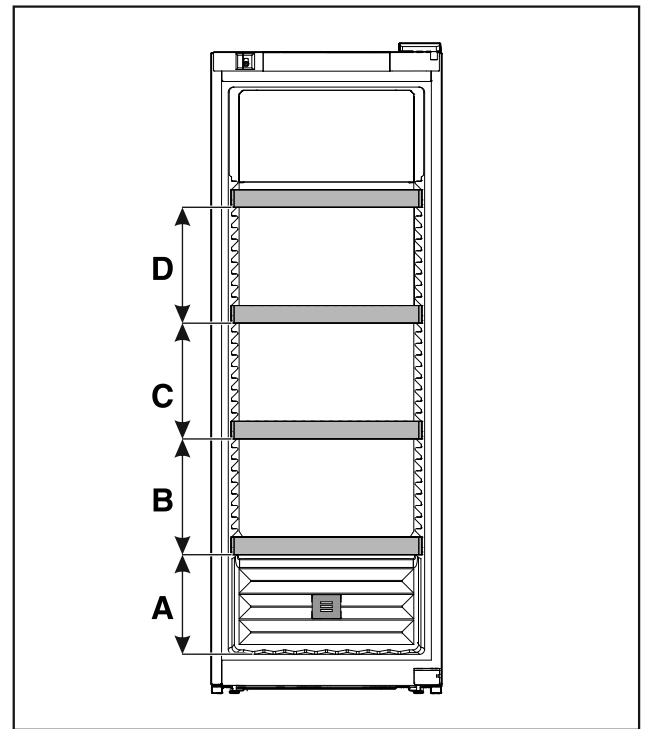
Fig. 12 Abstände Auflageroste
