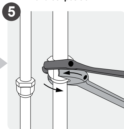
Rohre anschließen
