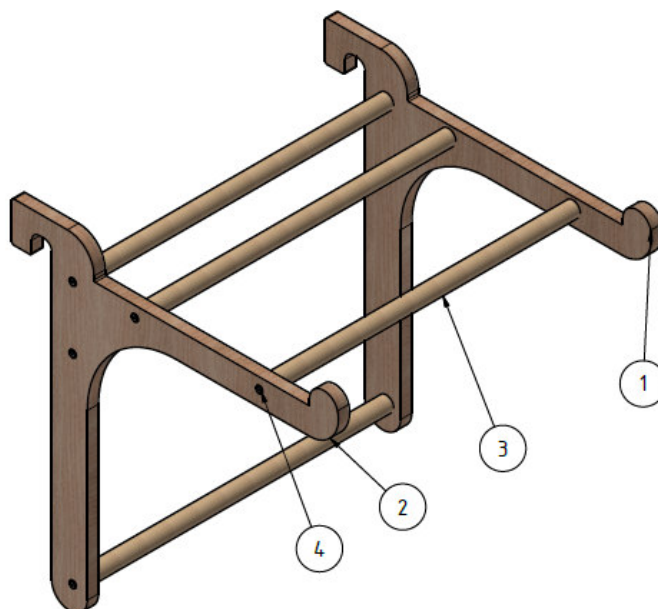
Abbildung 2: Multibügel "Wood"
