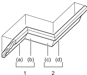
1. Innenecke 2. Außenecke
