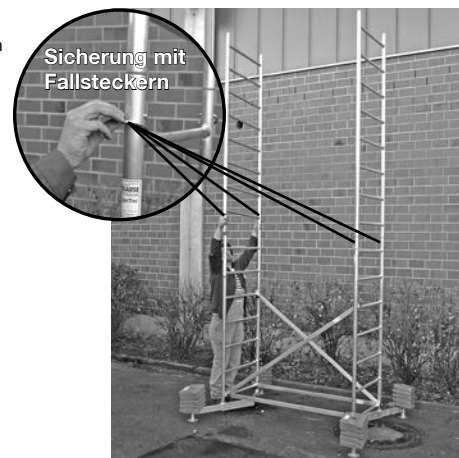
Grundgerüst mit erster und zweiter Aufstockung
