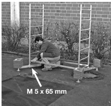
Grundgerüst mit erster und zweiter Aufstockung
