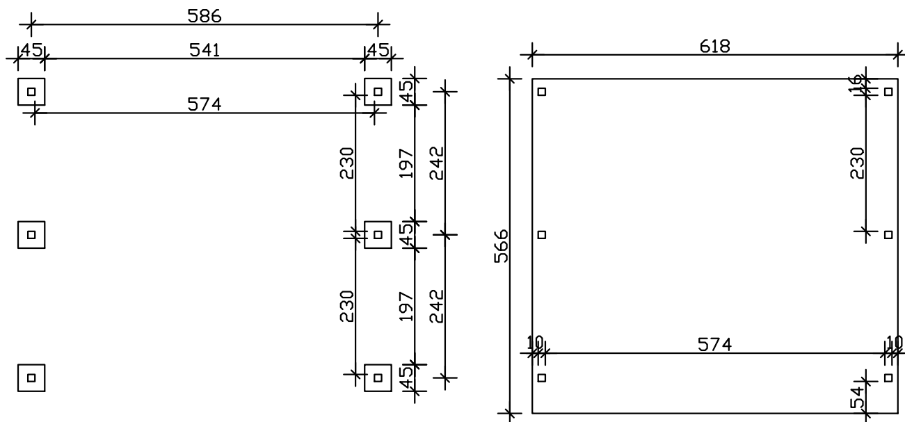
Grundriss
