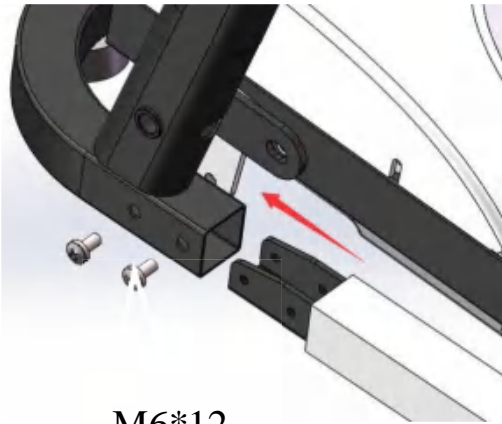
M6*12
