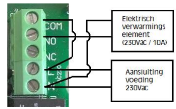
TBV Elektroheizung
