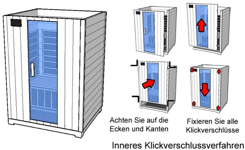
Bild C5: Türpaneel
