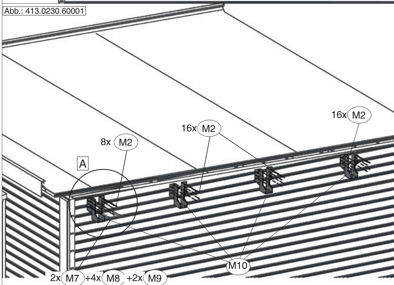
Abb.: 413.0225.60001
