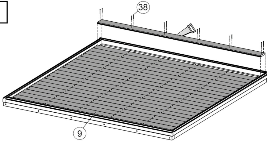
Abbildung Art.-Nr.: 413.2525
