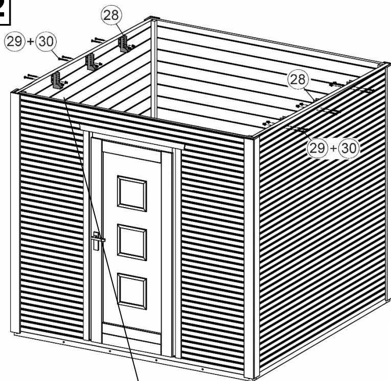
Abbildung Art.-Nr.: 413.2525
