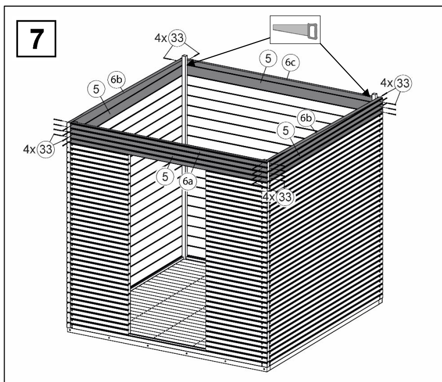
Abbildung Art.-Nr.: 413.2525
