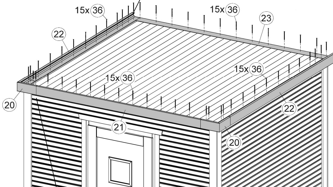
Abbildung Art.-Nr.: 413.2525
