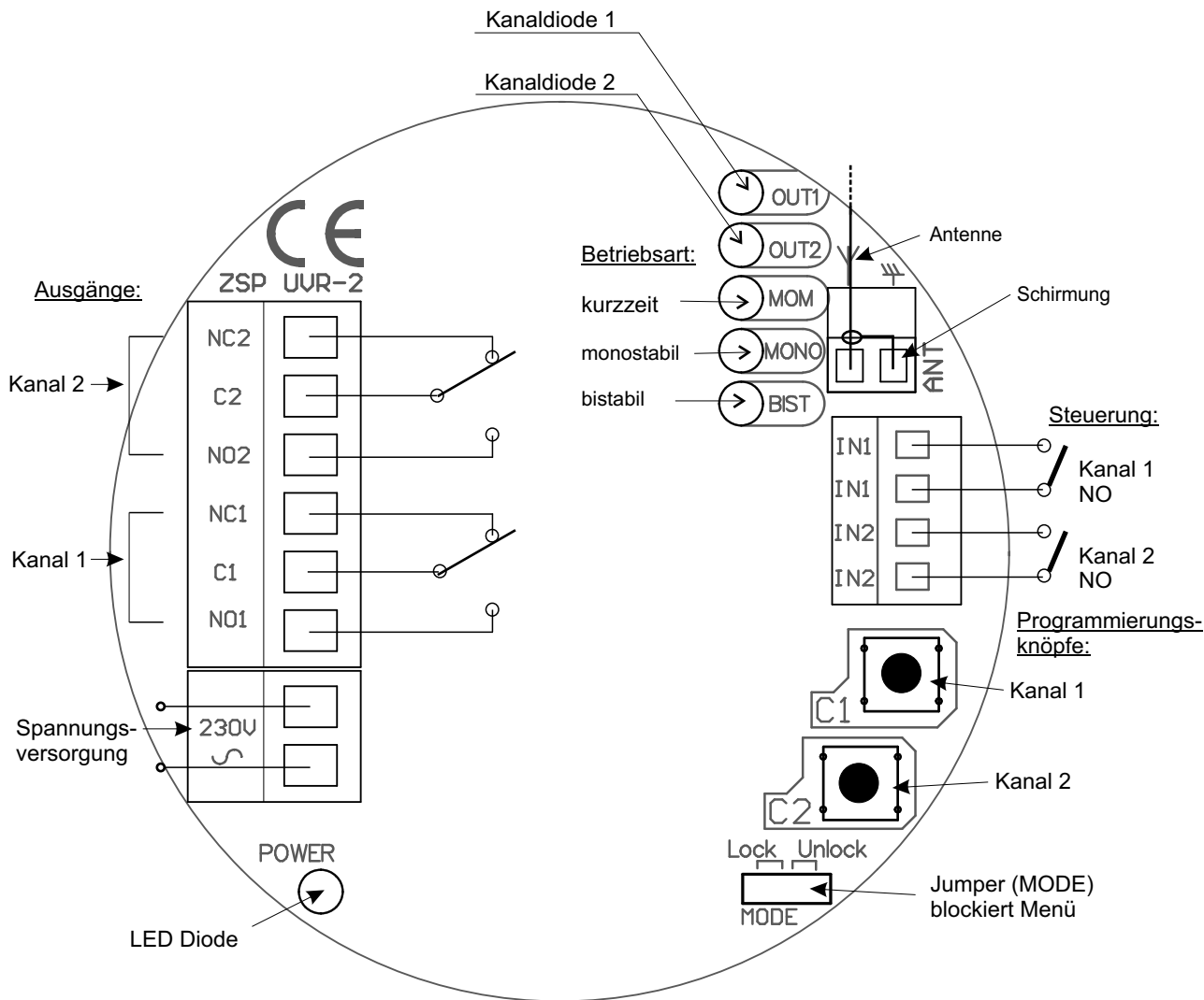
Abb. 1 Elektrische Verbindungen Empfänger Universal (UVR-2)
