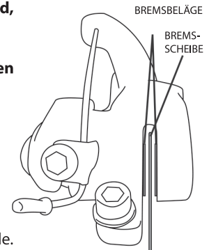
BREMSSSCHEIBE
