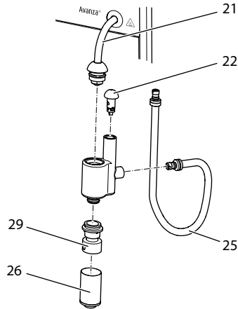
Fig. 15: Demontere Cappuccinatore
