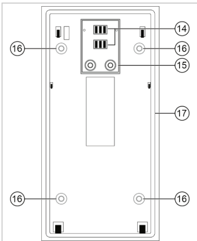
Montageplatte
