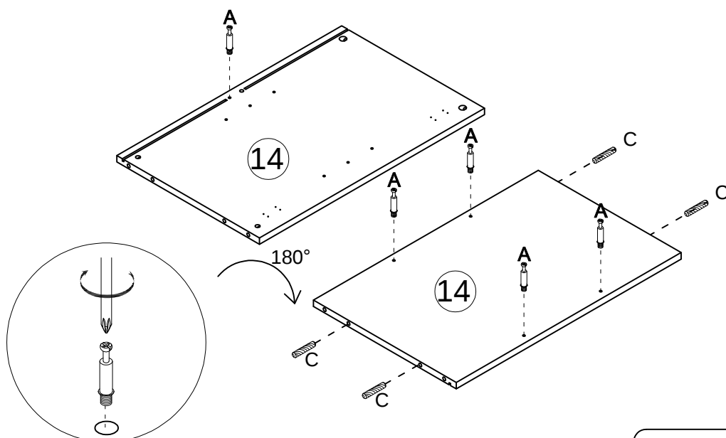
eccentric rod
