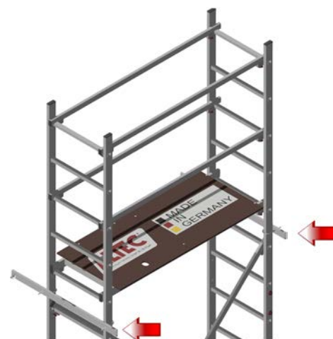
Position der Wandverankerungen
