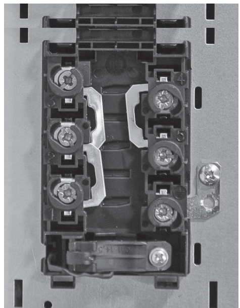
Anschlussbox geöffnet
